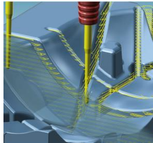
Software „HyperMill“
