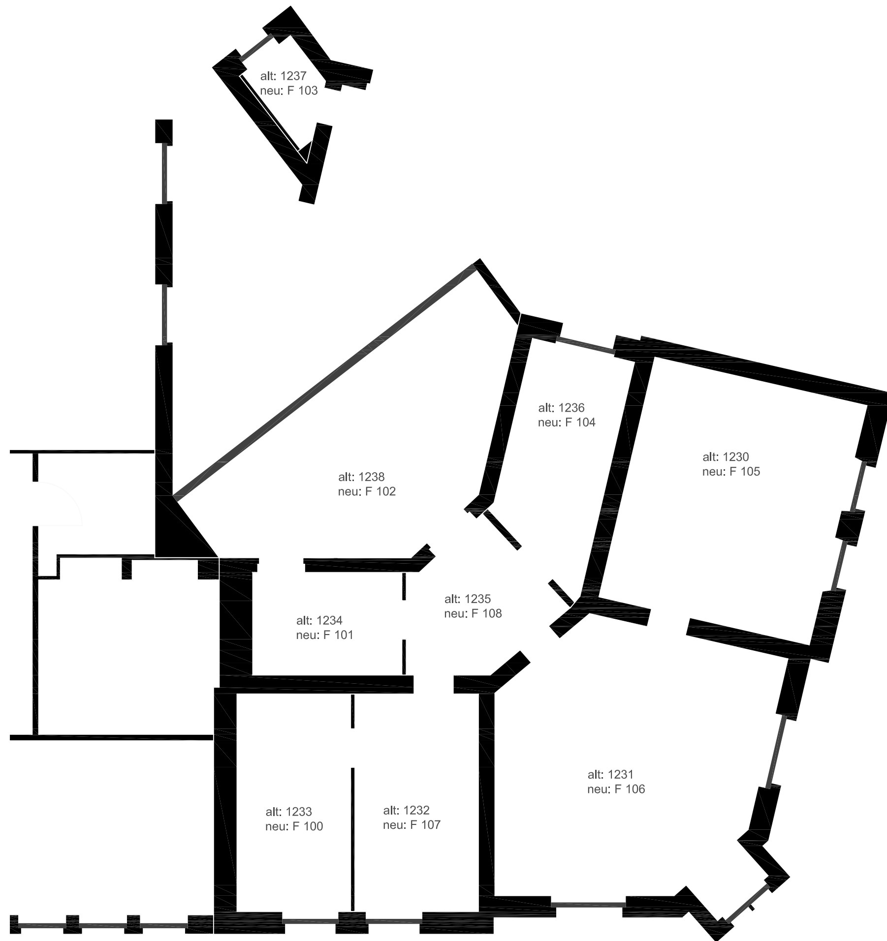
Gebäude F 1. Obergeschoß
