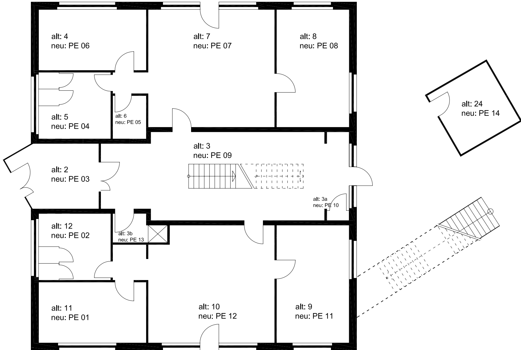
Gebäude P Erdgeschoss
