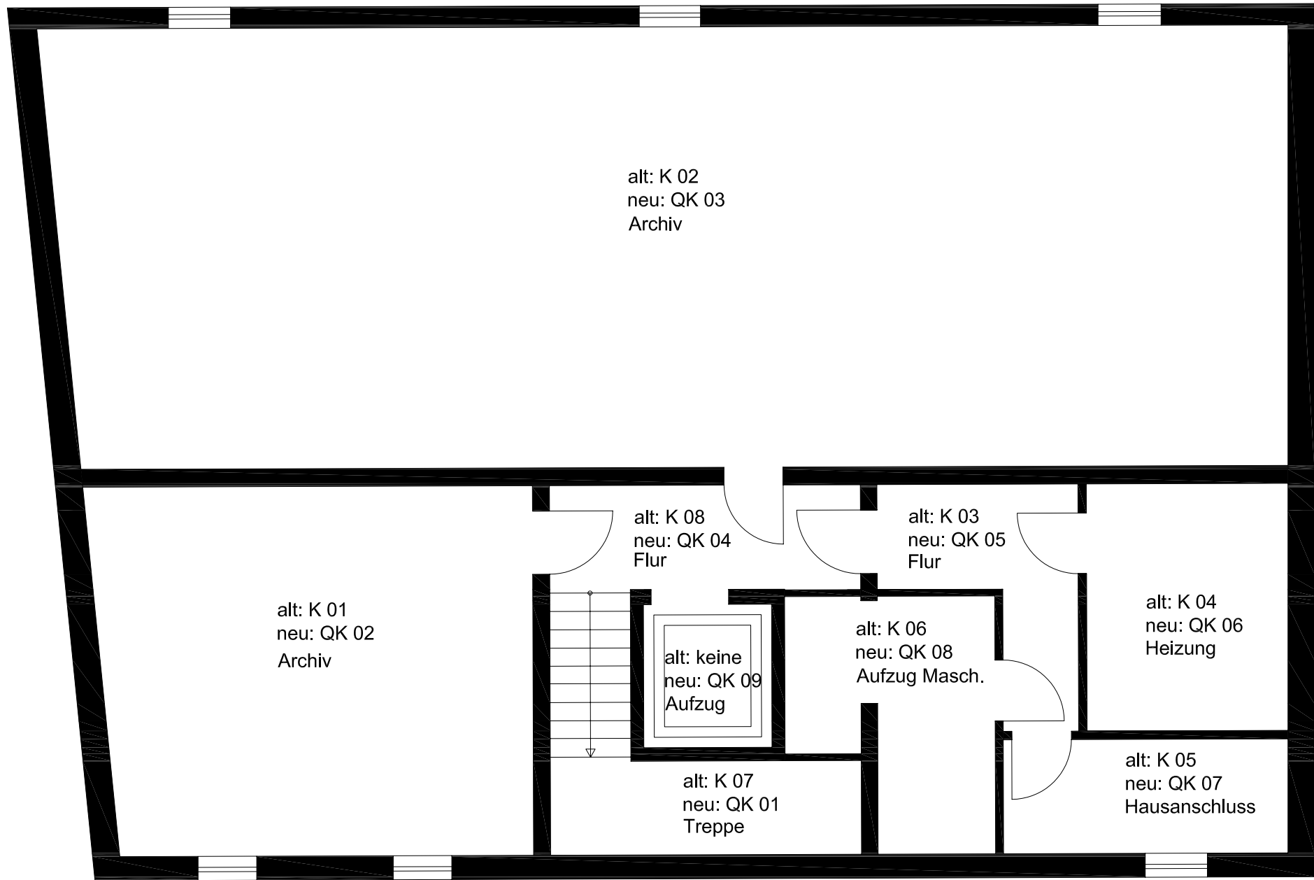
Gebäude Q Kellergeschoss
