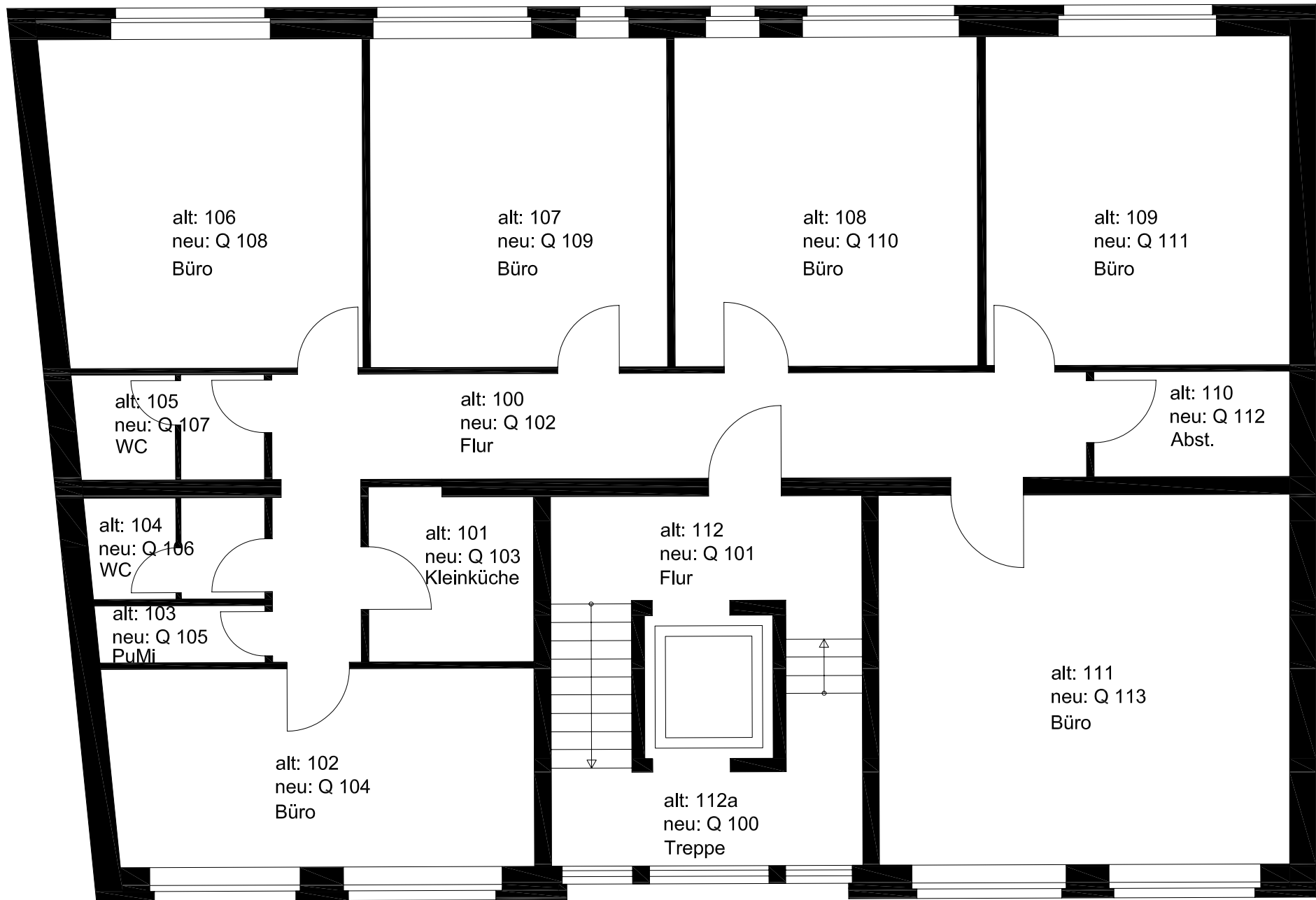
Gebäude Q 1. Obergeschoss
