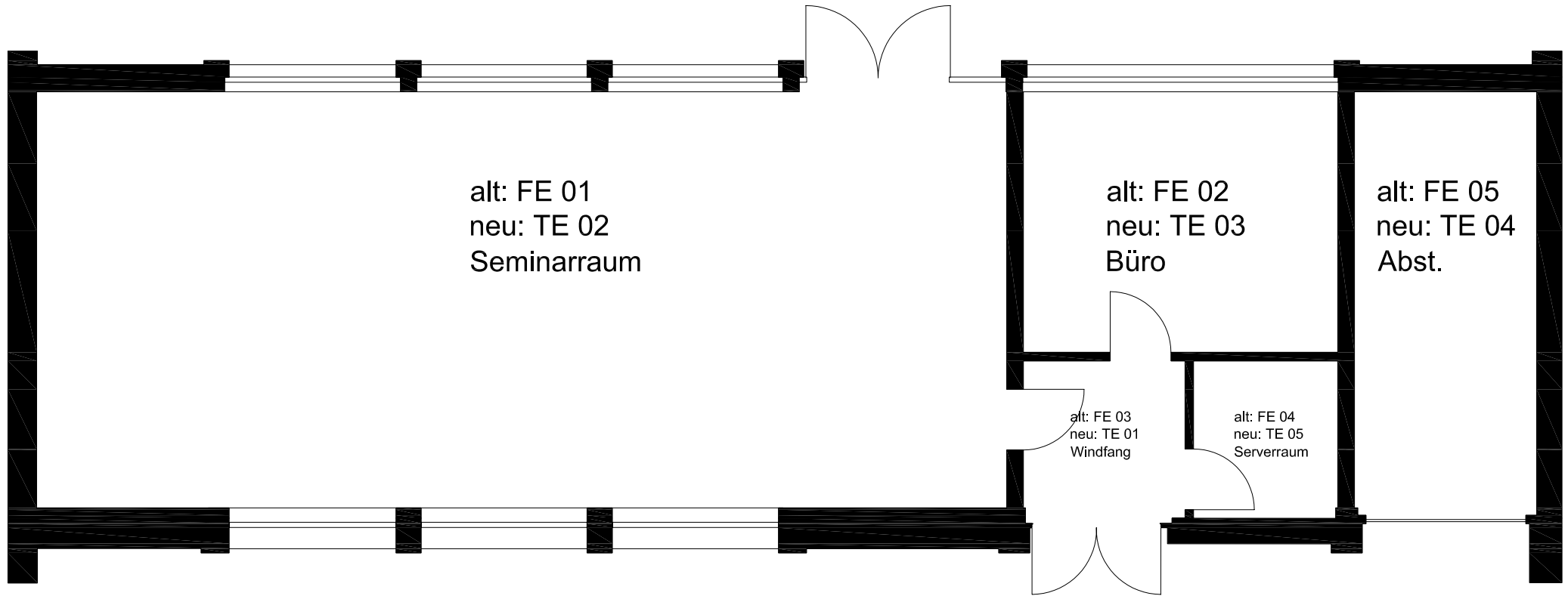
Gebäude T Erdgeschoss
